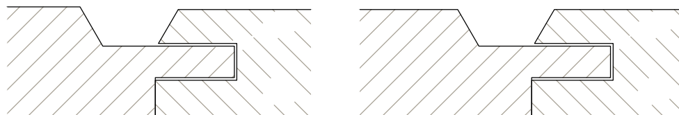
Samledetalje / Verbindungsdetail
