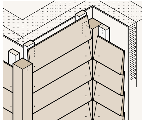
Indvendig hjørneløsning
