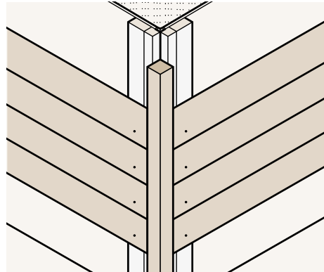
Udvendig hjørneløsning
