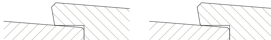
Samledetalje / Verbindungsdetail
