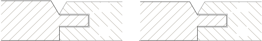
Samledetalje / Verbindungsdetail
