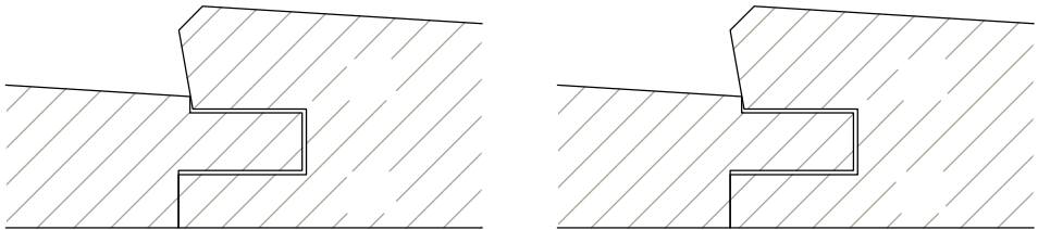
Samledetalje / Verbindungsdetail
