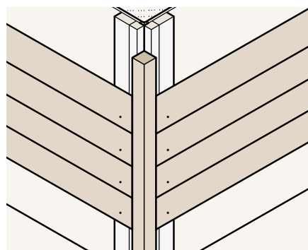
Udvendig hjørneløsning
