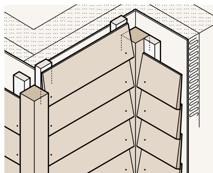
Indvendig hjørneløsning
