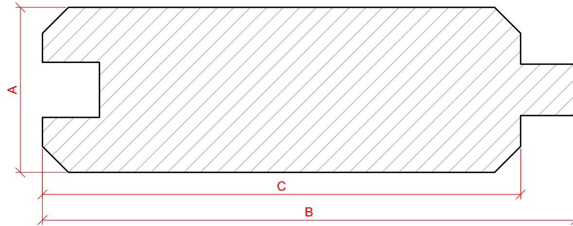
Samledetalje / Verbindungsdetail
