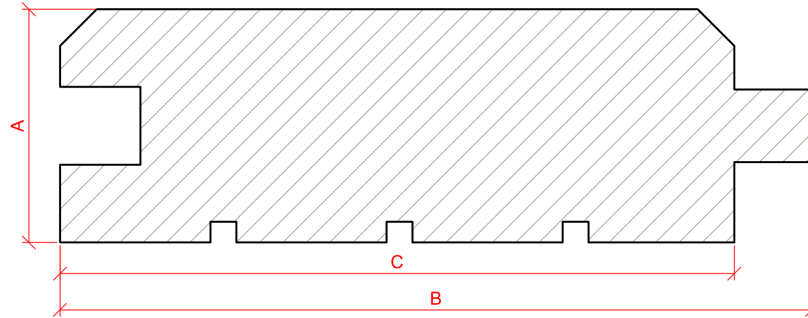
Samledetalje / Verbindungsdetail
