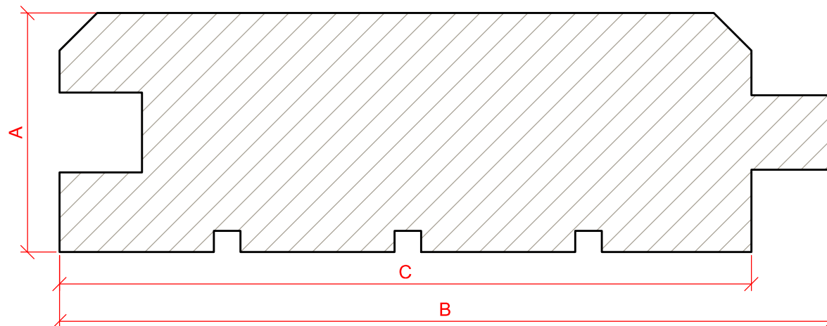
Samledetalje / Verbindungsdetail
