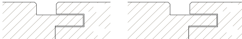
Samledetalje / Verbindungsdetail
