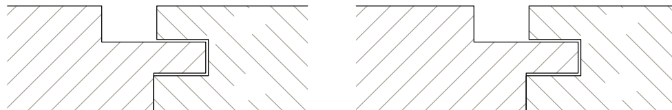
Samledetalje / Verbindungsdetail
