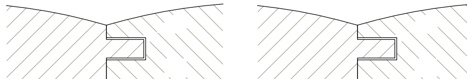
Samledetalje / Verbindungsdetail
