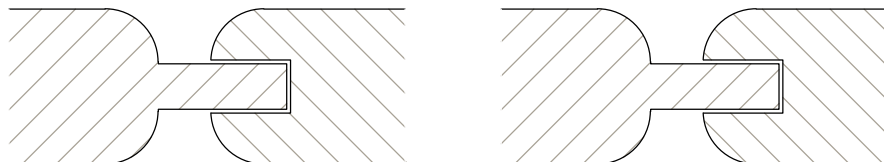
Samledetalje / Verbindungsdetail
